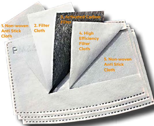
5 LAYER CONSTRUCTION
